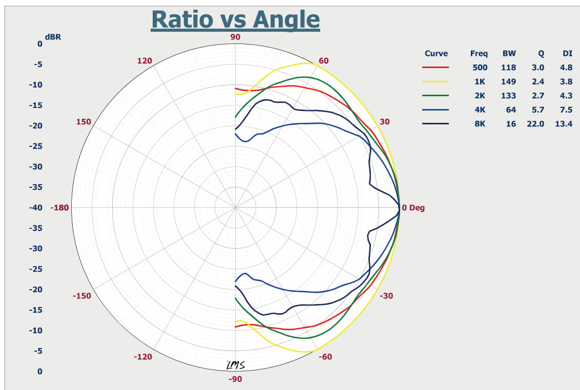
Круговая диаграмма направленности громкоговорителя LPA-10C
